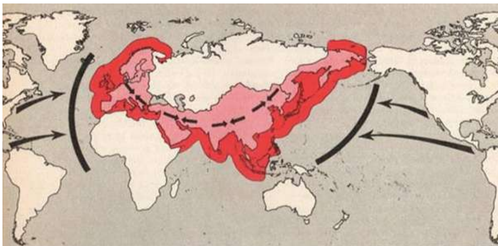
Le Rimland et les mers marginales entourant le continent. Carte de Spykman 10 .
